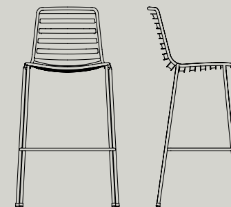
Stool W565 H1 1090 H2 990 D530
